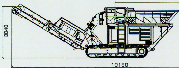
Pracovní poloha
